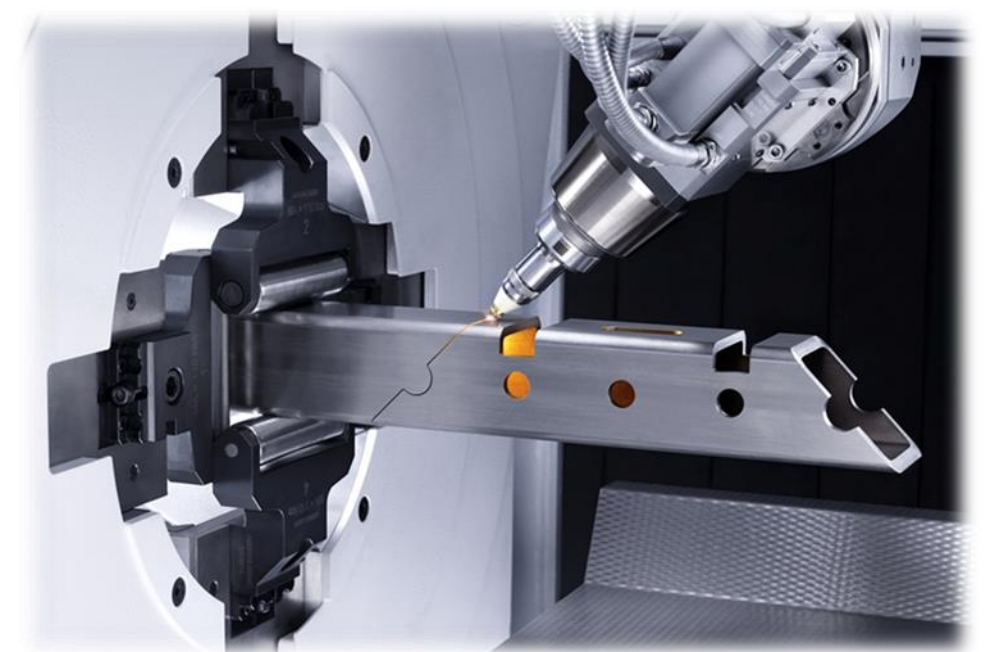
雕花開孔、折彎、接口接合實例
